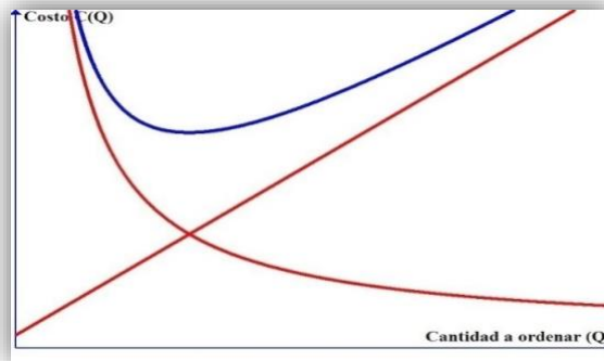
Figura 3. Gráfica del COSTO TOTAL del modelo EOQ
