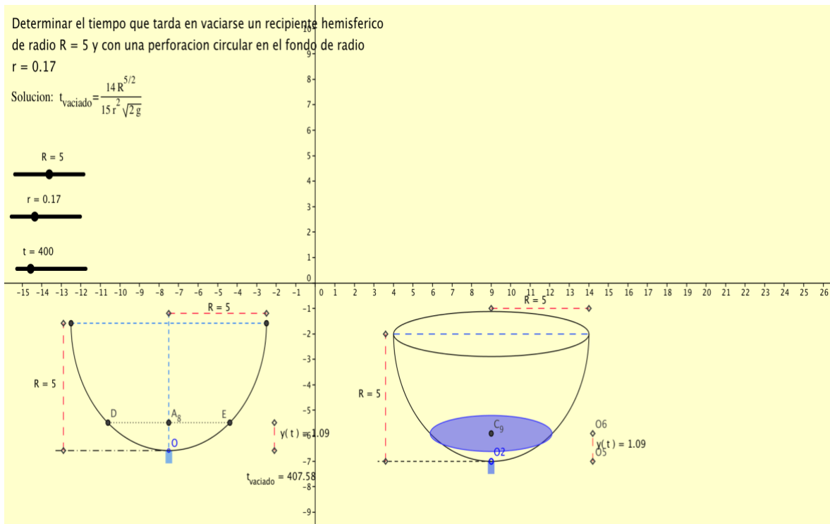
Fig. 7 Fase terminal del vaciado de recipiente
