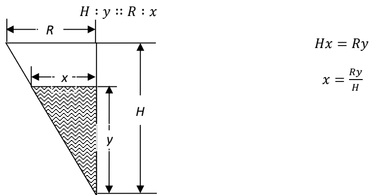
Fig. 3 Sección del depósito con dimensiones x , y .
